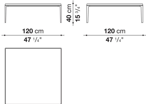
MT120Q
