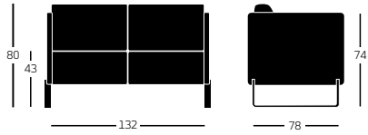
Ref: 572S Sofá bajo tapizado. Pies pletina / Upholstered sofa. Sheet steel legs.
