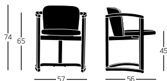
Ref: 380 Silla en laminado de haya. Fija / Beech laminated frame. FIX armchair.
