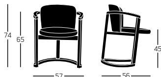
Ref: 381 Silla en laminado de haya. Balancín / Beech laminated frame. ROCKING armchair.
