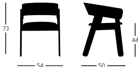
Ref: 515T Estructura de haya. Asiento tapizado / Beech wood. Upholstered seat.
